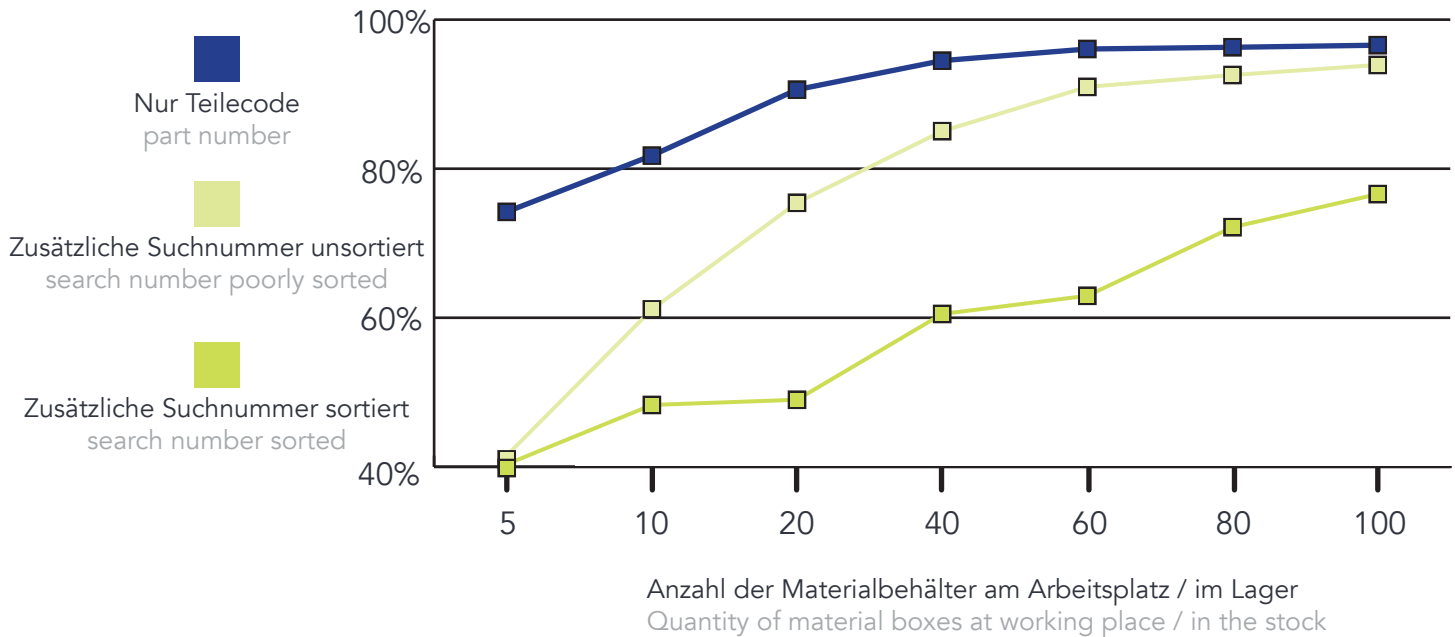
Durchschnittliche Zeitersparnis bei der Materialsuche mit pick-to-light Average time saving during material search with pick-to-light
